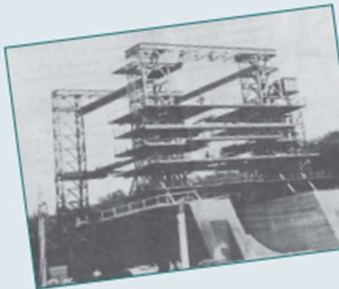
Triebwerksprüfstand Bild: © Militärarchiv Freiburg
